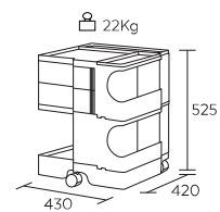
2段2トレイ
