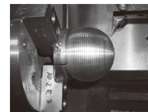
旋盤加工
