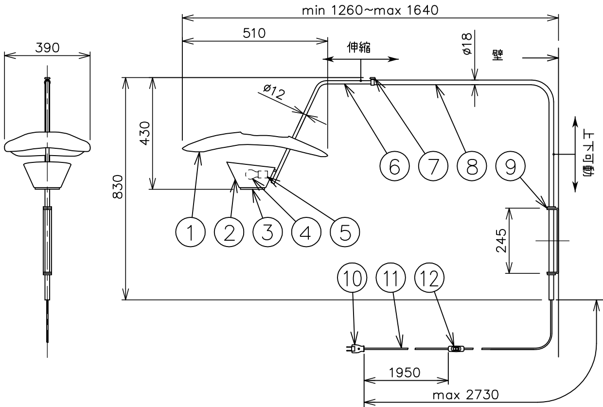
取付面図
