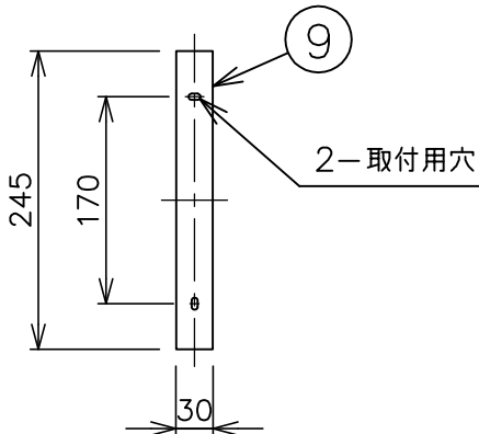
取付面図
