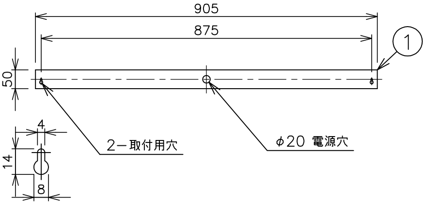
取付面図
