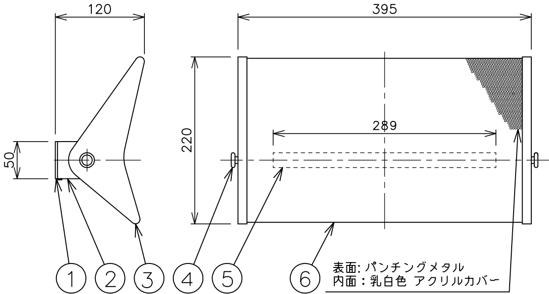
取付面図
