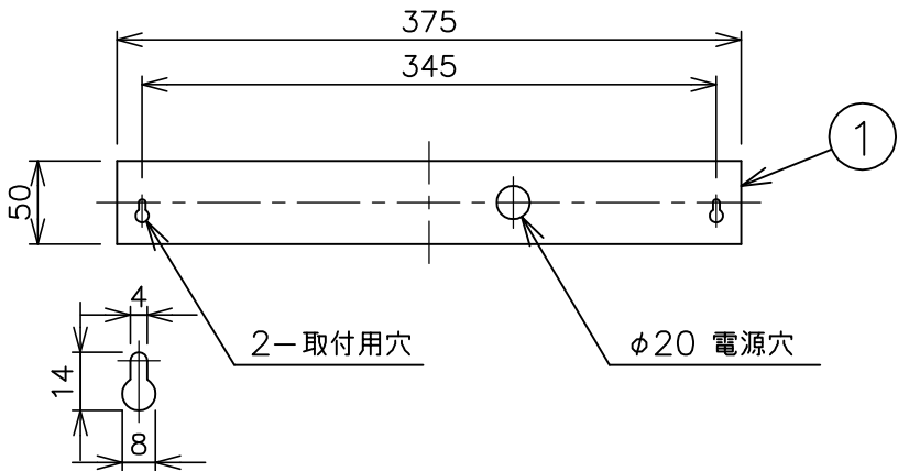
取付面図
