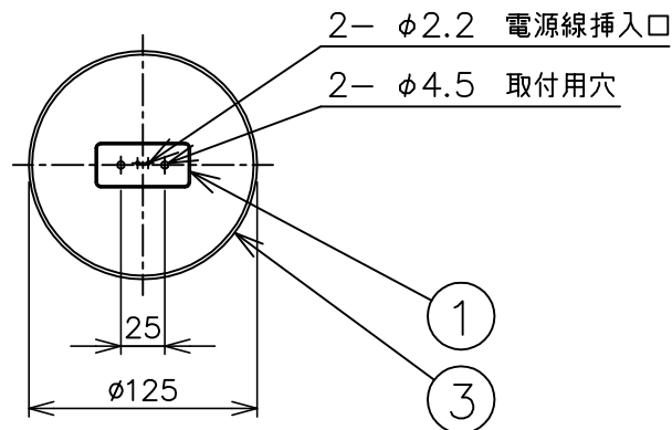
取付面図
